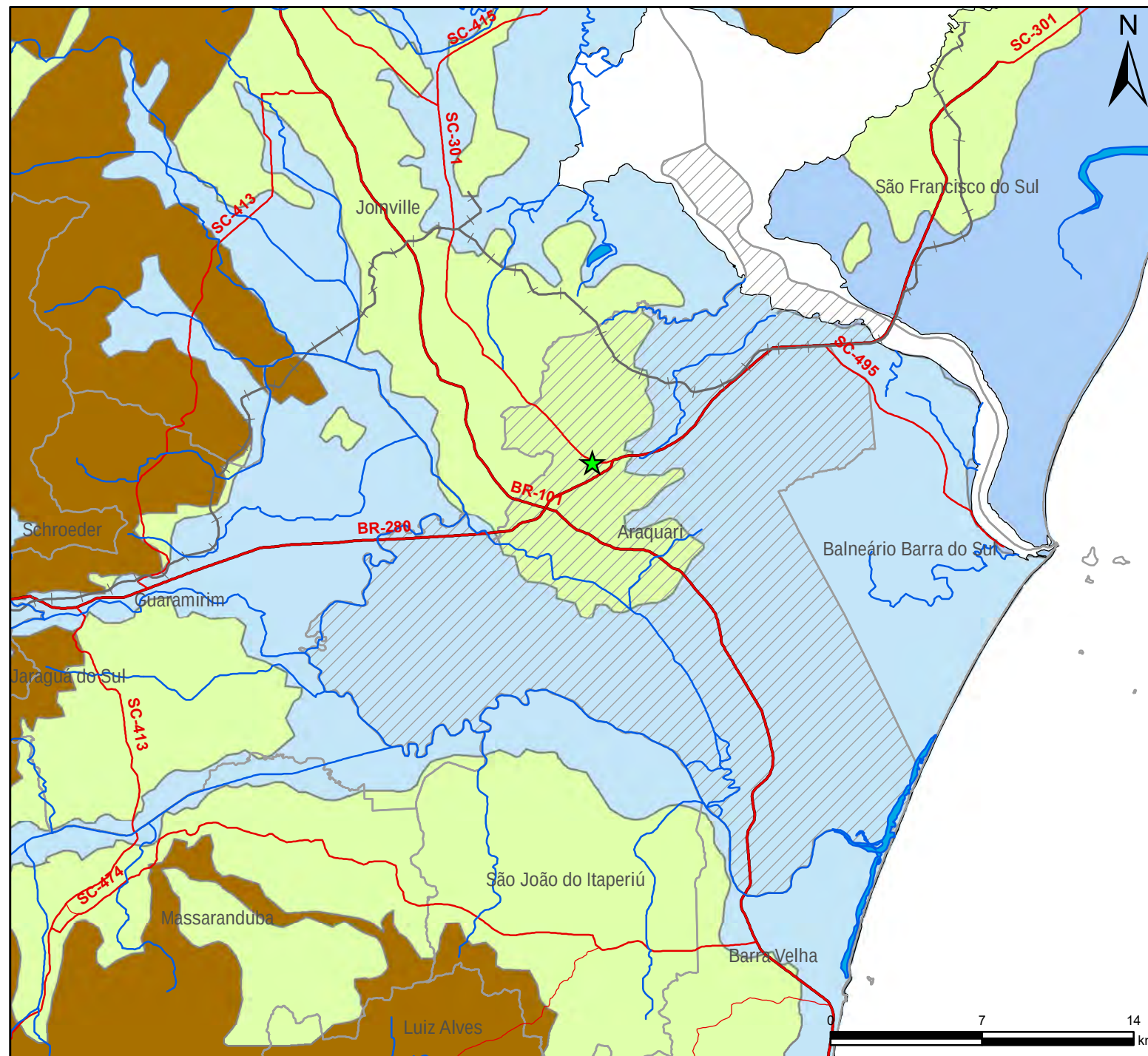
Figura 3. Mapa Hidrogeológico Regional
