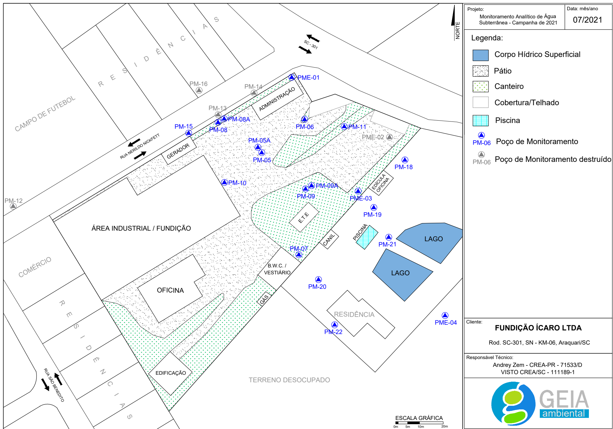
Figura 4. Planta baixa e localização dos poços preexistentes
